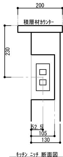
キッチン ニッチ 断面図
